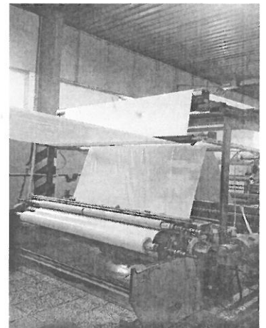
Extrudovanie fólie
